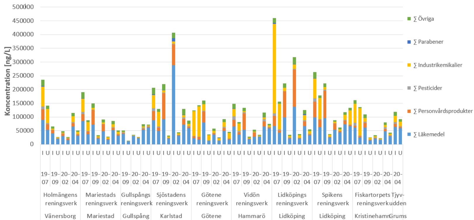
Figur 30. Kumulativa koncentrationer av de studerade organiska miljöföroreningarna, exklusive PFAS-ämnen, i deltagande avloppsreningsverk kring Vänern, med generella klassificeringar. Generaliserad bild av Figur 5. Datum enligt ÅÅ-MM. I: Inkommande, U: Utgående.
