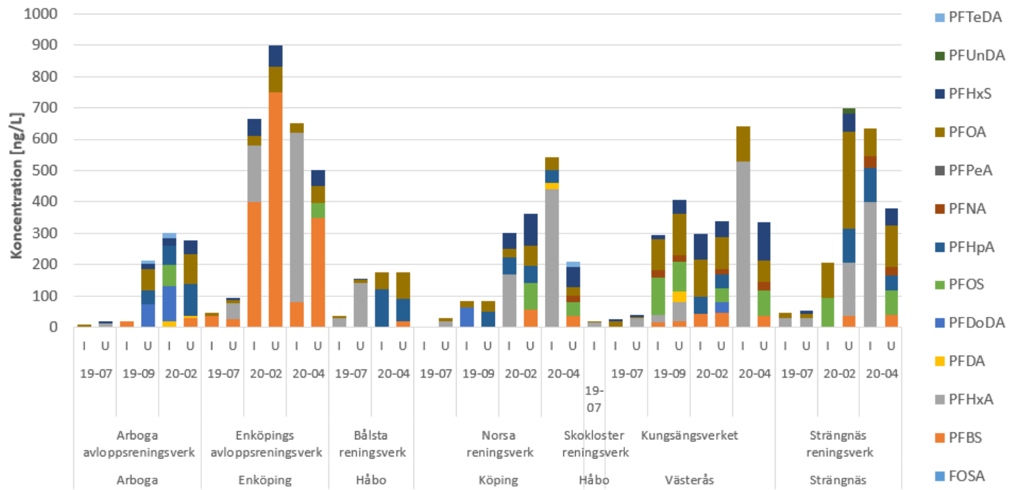
Figur 27. Kumulativa PFAS-koncentrationer i avloppsreningsverk kring Mälaren. Datum enligt ÅÅ-MM. I: inkommande avloppsvatten, U: utgående avloppsvatten
